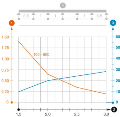
Diagramme de charge échelle à câbles type SLZ ALU
