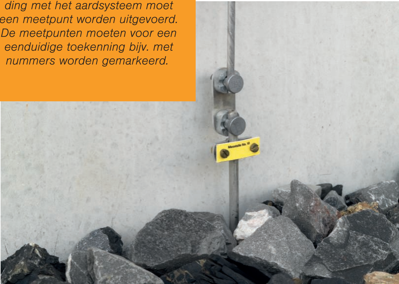
Meetpunt op de aarde-invoer
