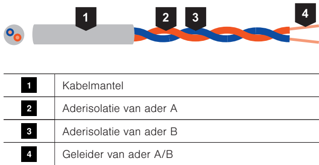
Symmetrische leiding
