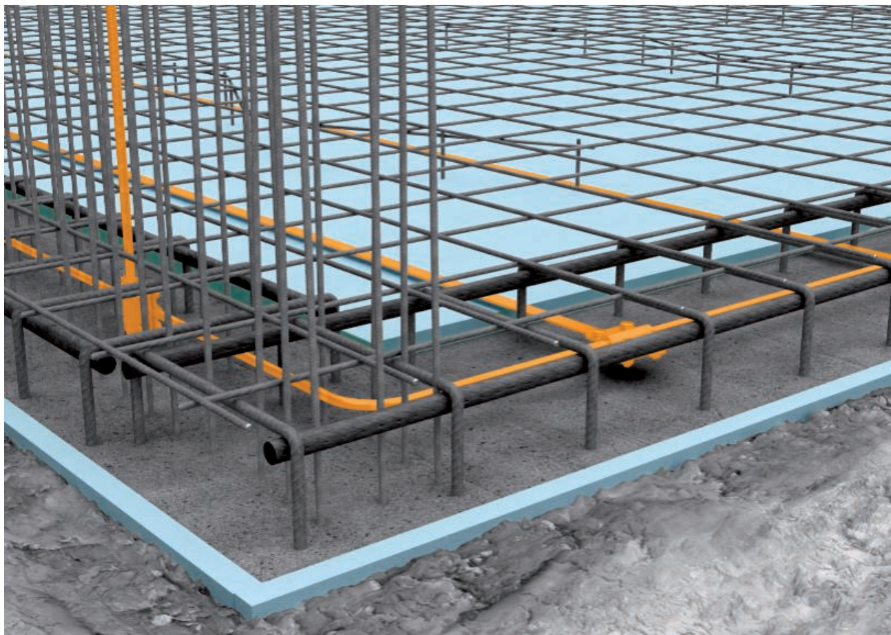
Geïsoleerde vloerplaat (perimeterisolatie, hier: blauw)
