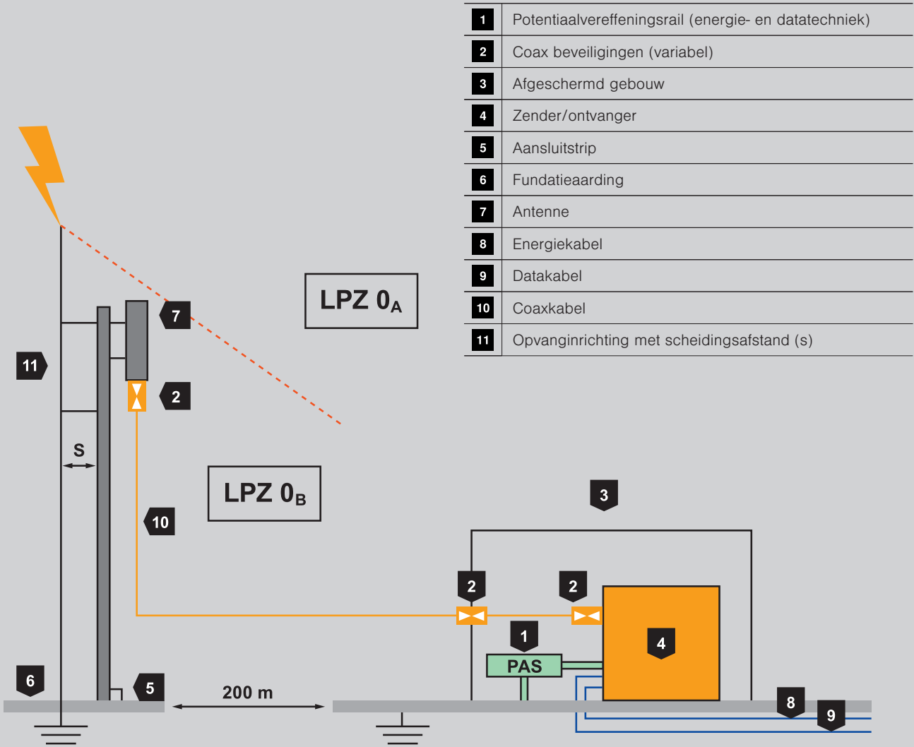
Geïsoleerde bliksembeveiliging op antennesysteem en verschillende aardingssystemen
